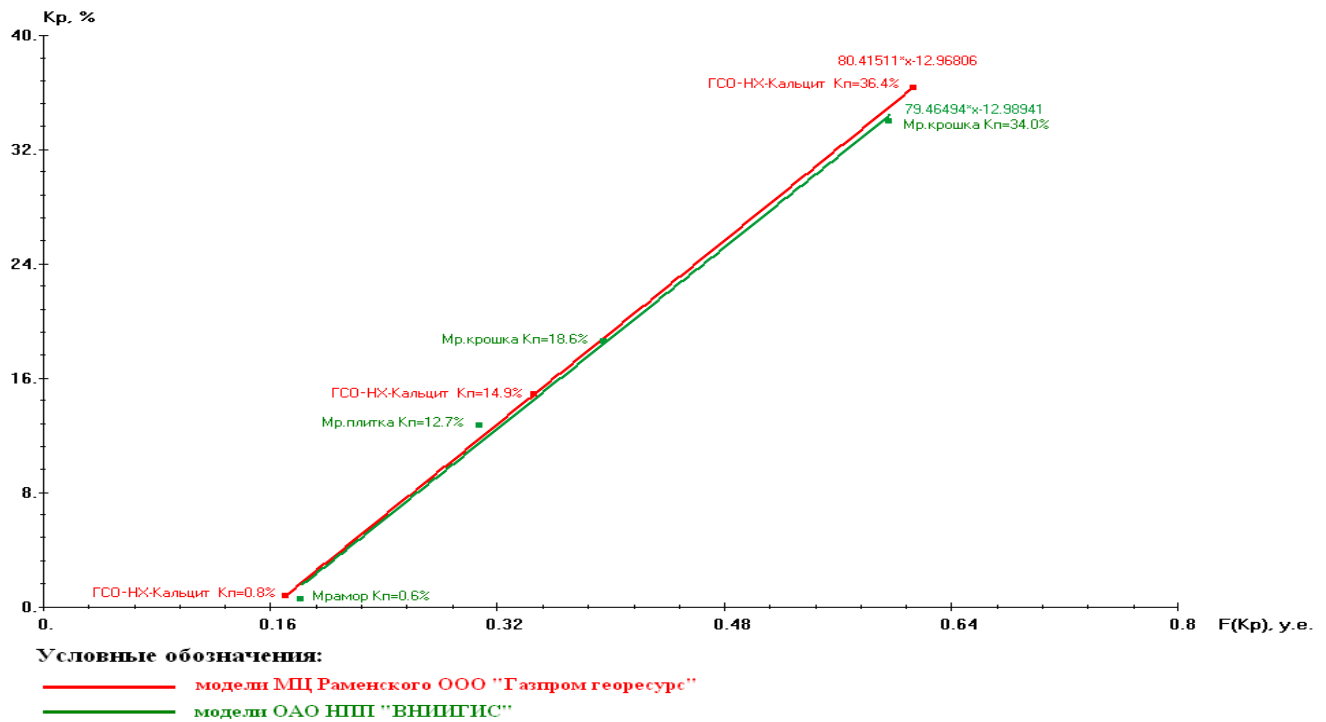
Рис. 4.2 Сопоставление основных зависимостей Kп = F(Kп) для метода 2ННК на моделях пластов известняка, насыщенных пресной водой, в скважинах диаметром 200 мм, заполненных пресной водой, выполненных в метрологических центрах ОАО НПП «ВНИИГИС» и ООО «Газпром георесурс». Прибор центрирован в скважине
