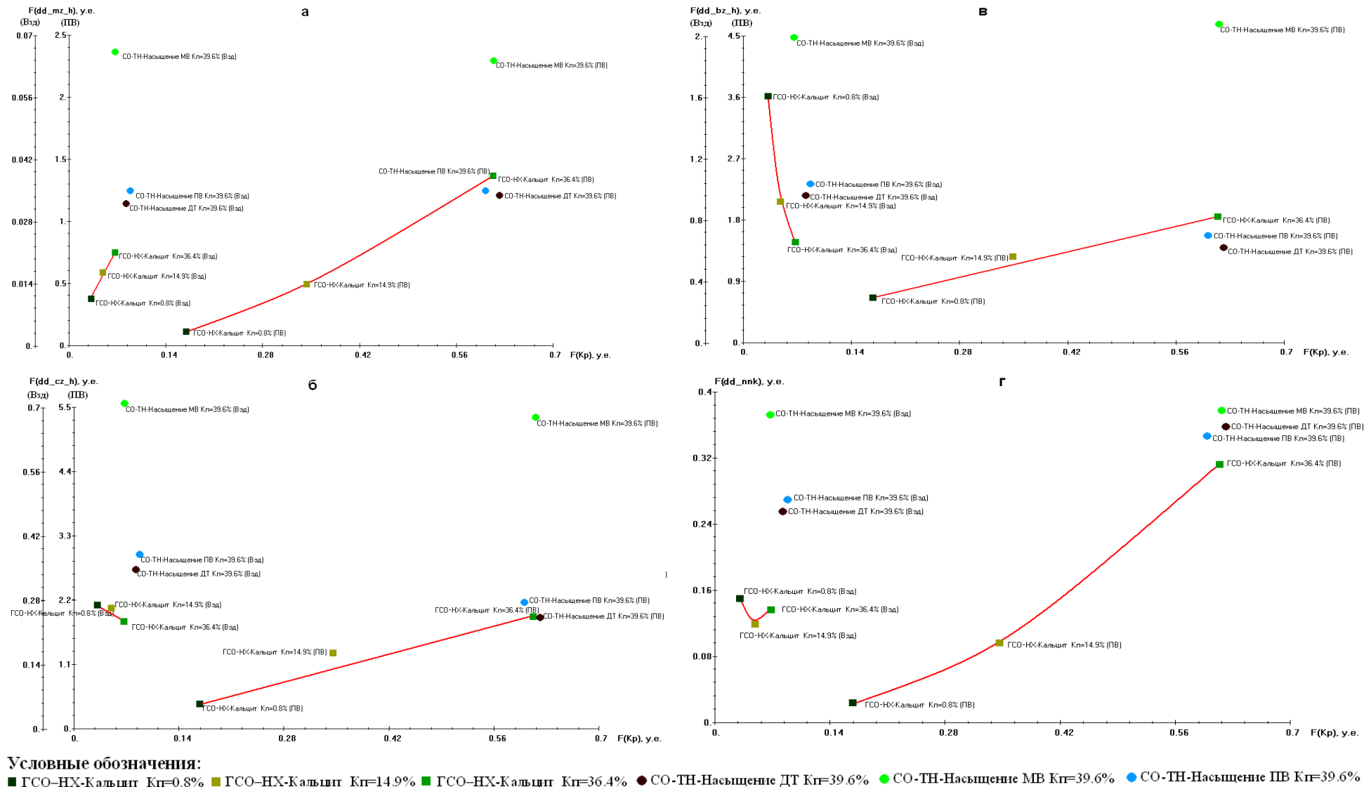
Рис 4.4 Экспериментальные зависимости вычисленных функций характера насыщения F(n) от F(Kn) , выполненных на моделях пластов ООО «Газпром георесурс» для малого (а), среднего (б), большого зондов (в) СНГК и метода 2ННК (г)
