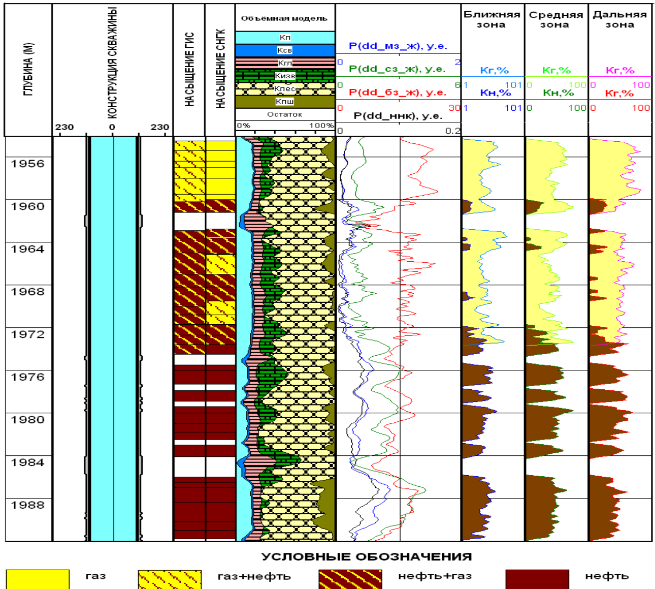
Рис. 5.9 Результаты интерпретации зондирования при-скважинной зоны комплексом разnogлубинных нейтронных методов с целью определения линейных размеров переходной зоны между нефтенасыщенным и газонасыщенным коллектором
