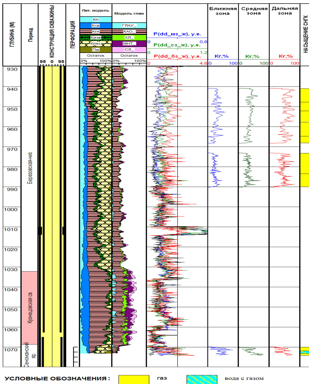
Рис. 5.13 Пример выделения нетрадиционных коллекторов по результатам зондирования в радиальном направлении разноточными нейтронными методами СНГК и ННК с вычислением K_2 – Березовская свита
