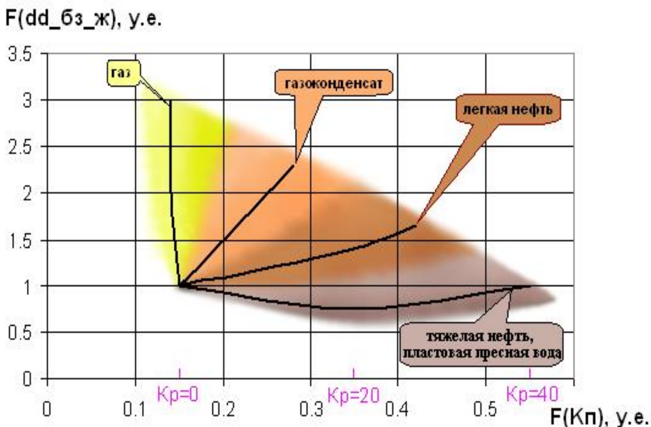
Рис. 5.4 Схема интерпретации функции дефицита плотности и водородосодержания F(dd\_бз\_ж) и функции пористости F(Kn) для определения фазового состава углеводородов в коллекторе при низкой минерализации пластовых вод
