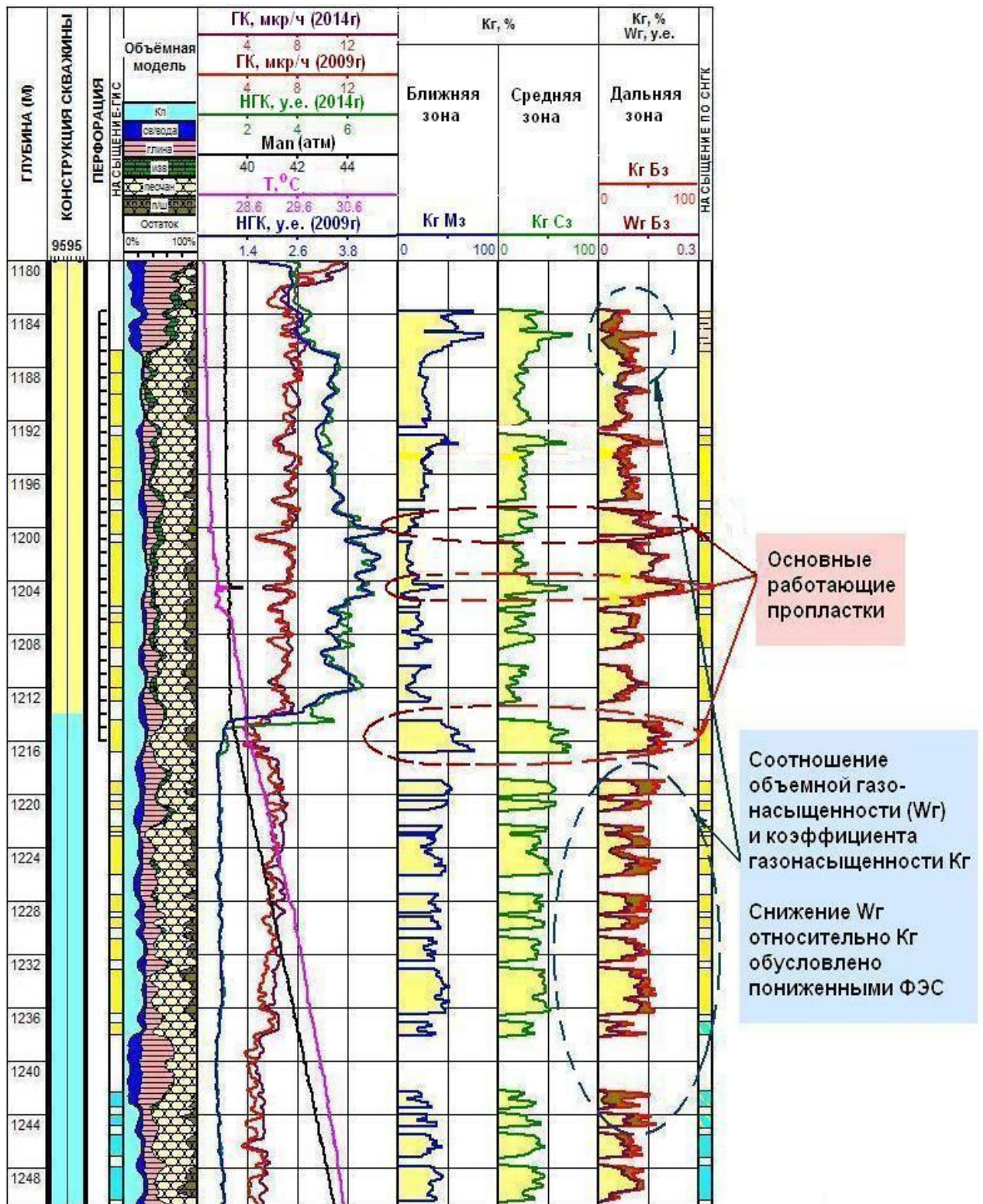
Рис. 5.8 Результаты обработки и интерпретации комплекса СНГК и ННК в перфорированном интервале газонаполненной скважины и нескрытом газонасыщенном интервале водонаполненной части скважины Уренгойского ГКМ
