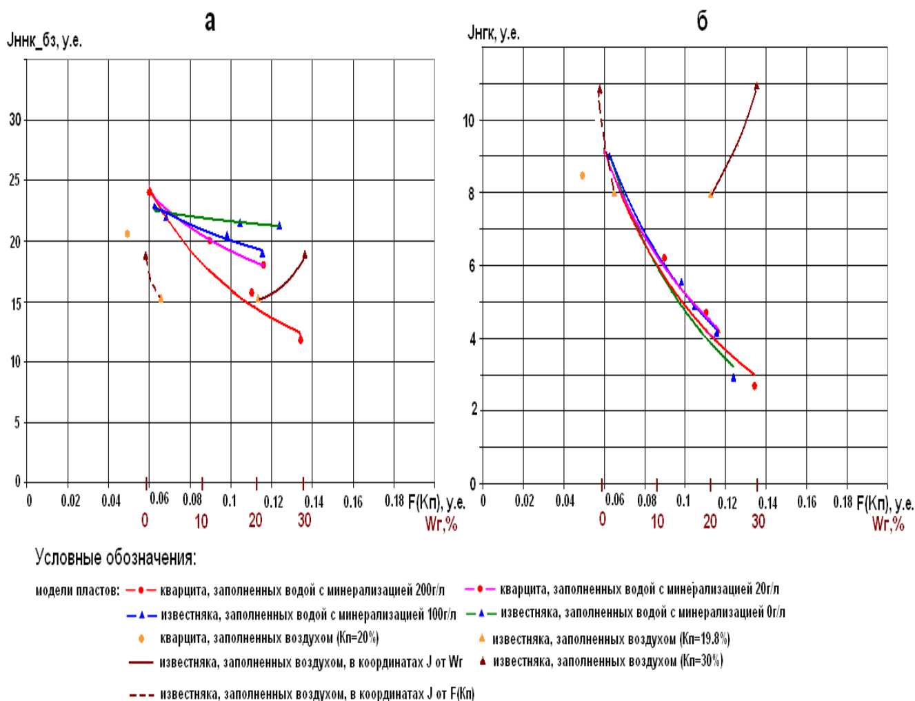
Рис. 3.6 Экспериментальные зависимости показаний методов ННК (а) и НГК (б) на больших зондах от функции пористости F(Kп) и объемного газонасыщения Wг при заполнении колонны диаметром 5" воздухом. Прибор диаметром 48мм центрирован в колонне, колонна центрирована в скважине, за колонной вода
